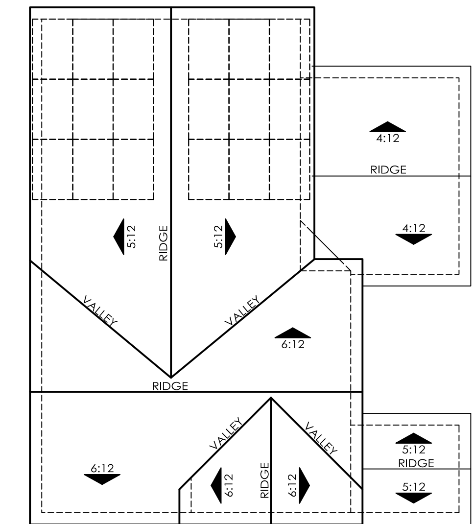
ROOF PLAN 5C OVERHANG : 12" RAKE : 12" ROOF PITCH : 6:12 U.N.O
