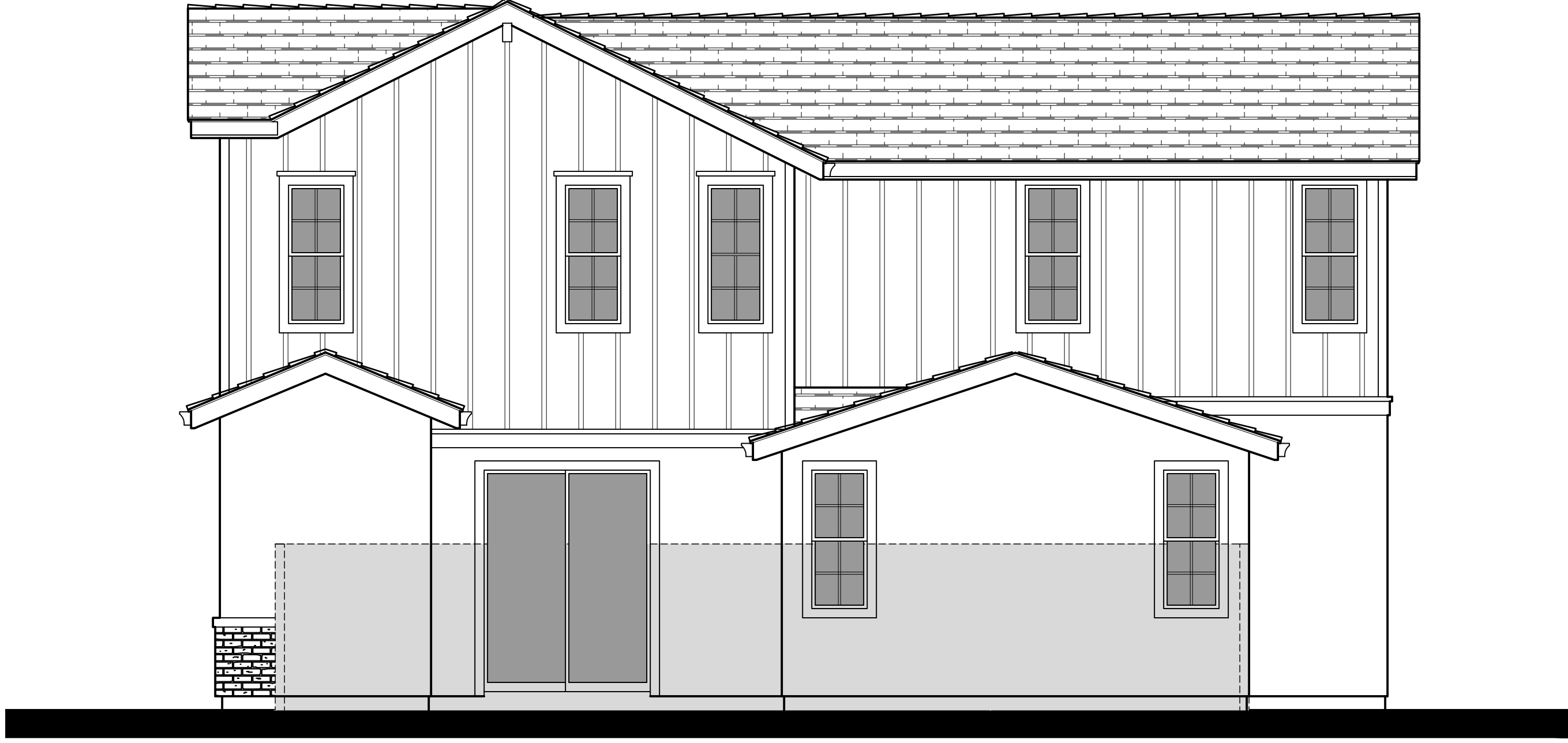
Right Elevation
