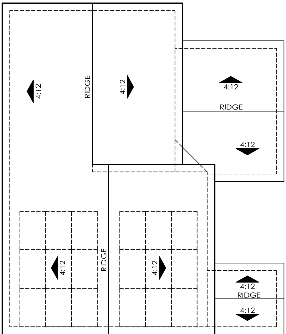
ROOF PLAN 5A OVERHANG : 12" RAKE : 12" ROOF PITCH : 4:12 U.N.O
