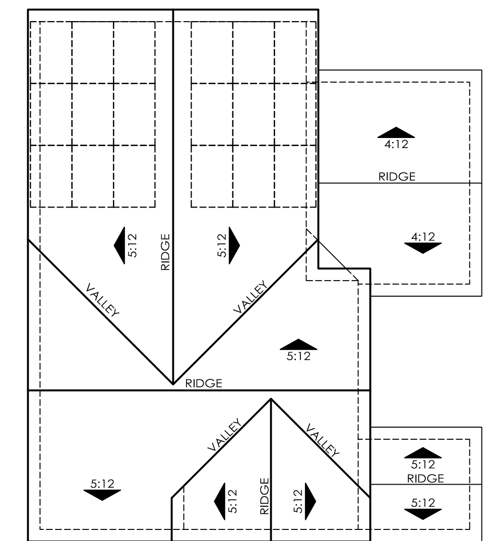
ROOF PLAN 5B OVERHANG : 12" RAKE : 12" ROOF PITCH : 5:12 U.N.O
